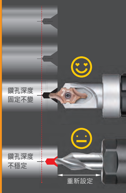
鎢鋼銑刀
